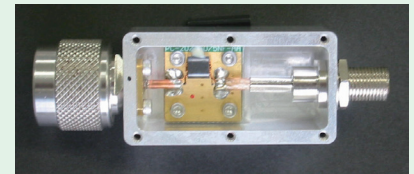
写真3:50Ω-75Ω変換器内部
